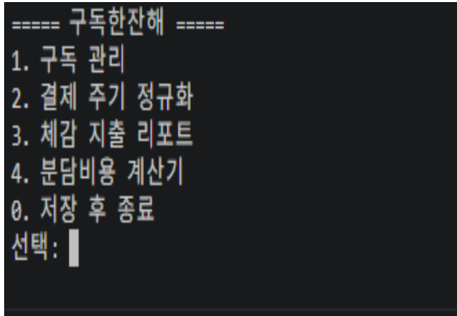
그림 3) 예상 콘솔화면
